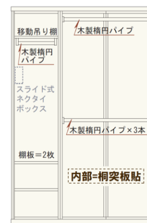
133スライド(3枚扉) W1335×D620×H2020
