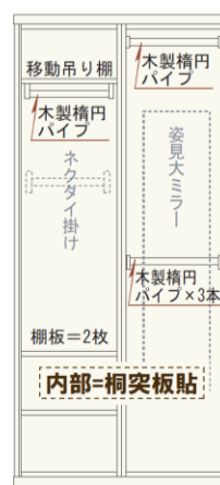
92プレザー(2枚扉) W922×D588×H2020
